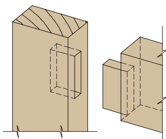
Blind Mortise & Tenon
